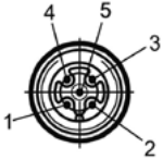
Plug (5 pol.)
