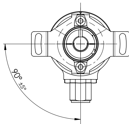
Frontansicht:
